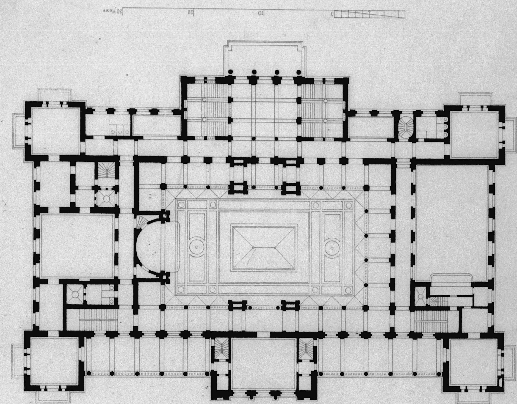
Grundriss des Hauptgeschosses
